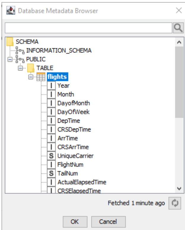
Figure 27. Database Metadata Browser
